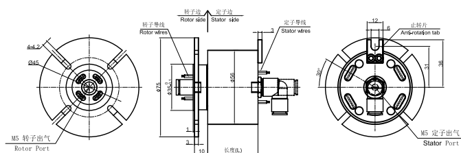
MAPH100-02 尺寸图
