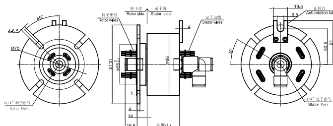
MAPH100-03 尺寸图
