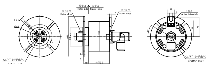
MAPH100-03 尺寸图
