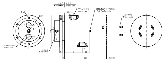
MAPH200-04 尺寸图
