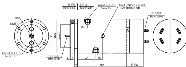
MAPH200-03 尺寸图
