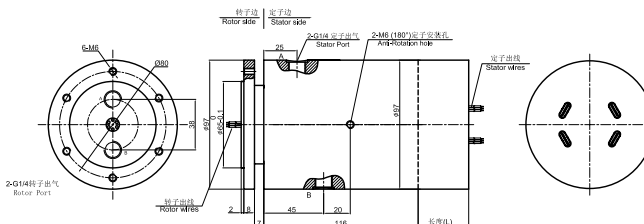
MAPH200-03 尺寸图
