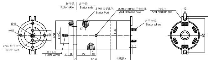
MAPH200-01 尺寸图
