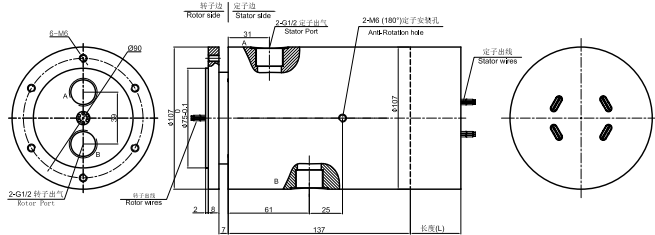
MAPH200-05 尺寸图
