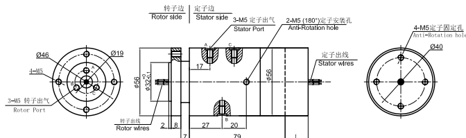
MAPH300S-02 尺寸图
