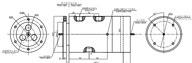
MAPH300S-05 尺寸图
