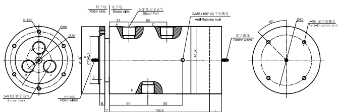
MAPH300S-05 尺寸图
