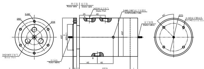
MAPH300S-03 尺寸图
