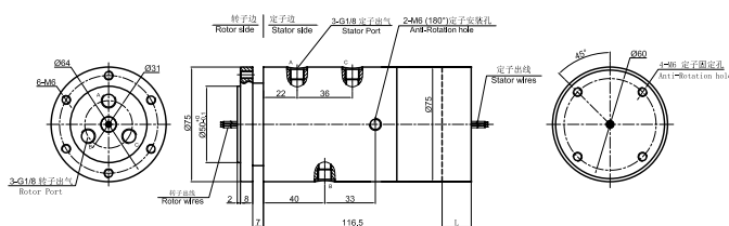
MAPH300S-03 尺寸图
