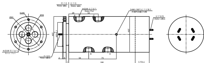
MAPH400-05 尺寸图
