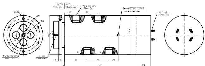
MAPH400-05 尺寸图
