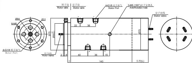
MAPH400-03 尺寸图
