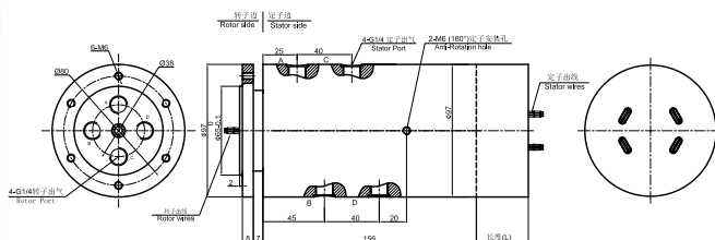
MAPH400-03 尺寸图
