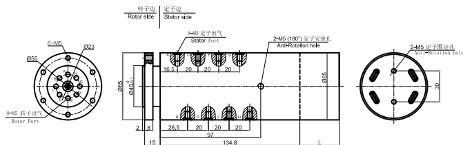
MAPH800-02 尺寸图
