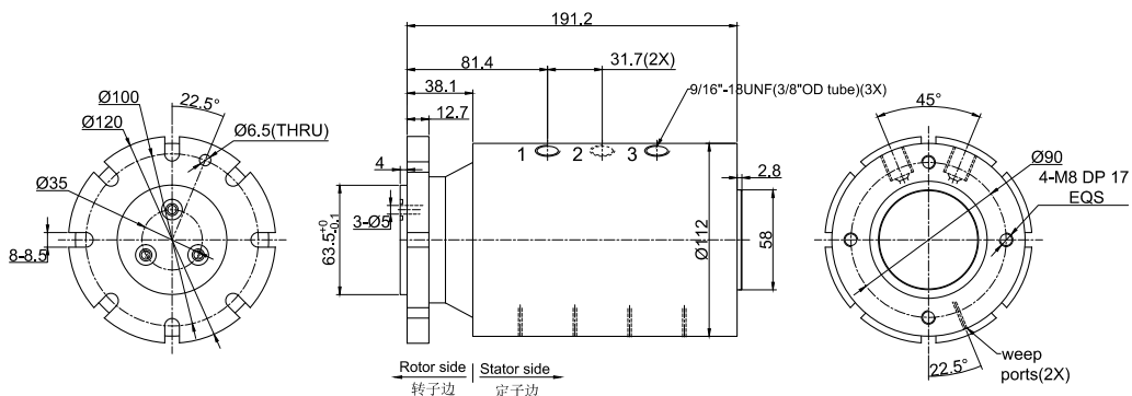
MHPS33 (高压不锈钢旋转接头) 尺寸图
