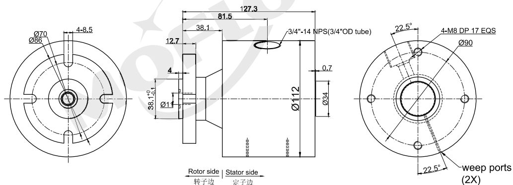
MHPS33 (高压不锈钢旋转接头) 尺寸图
