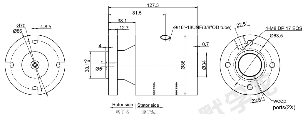
MHPS16 (高压不锈钢旋转接头) 尺寸图
