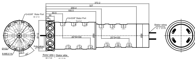
MK123-MT2586 尺寸图 12进12出G3/8"牙+信号(5A、10A)
