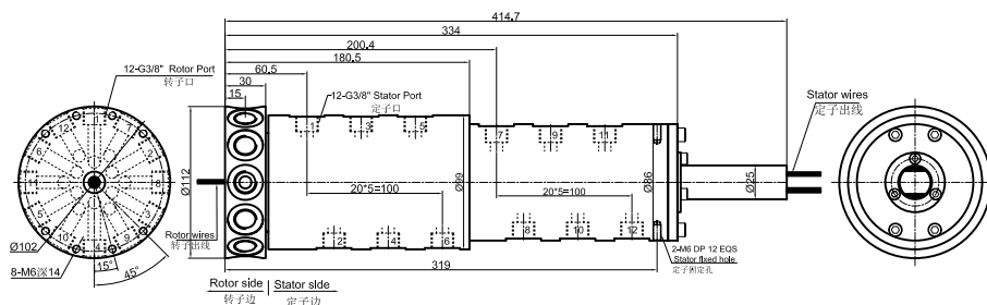
MK123S-S56 尺寸图 12进12出G3/8"牙
