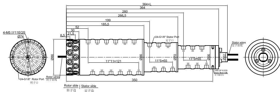
MK241S-S12(S18,S24,S36) 尺寸图 24进24出G1/8"牙+ 12~36路信号(2A)
