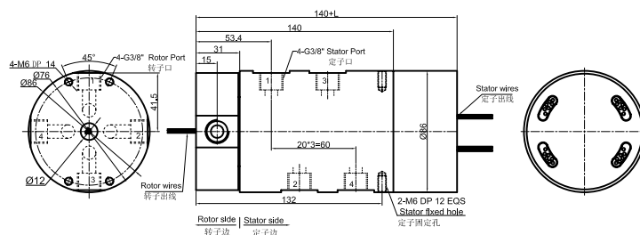
MK43-MT2586 尺寸图 4进4出G3/8"牙+信号(5A、10A)
