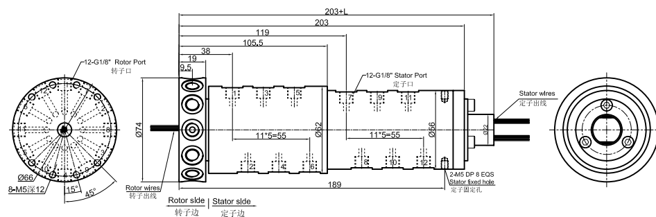
MK121S-S12(S18,S24,S36) 尺寸图 12进12出G1/8"牙+ 12~36路信号(2A)
