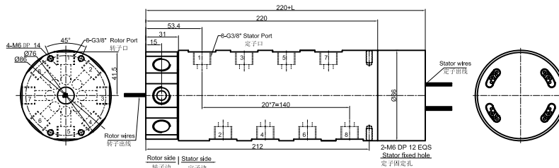
MK83-MT2586 尺寸图 8进8出G3/8"牙+信号(5A、10A)
