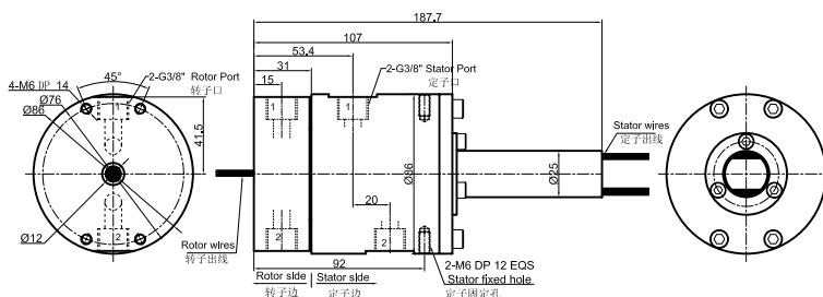
MK23S-S56 尺寸图 2进2出G3/8"牙
