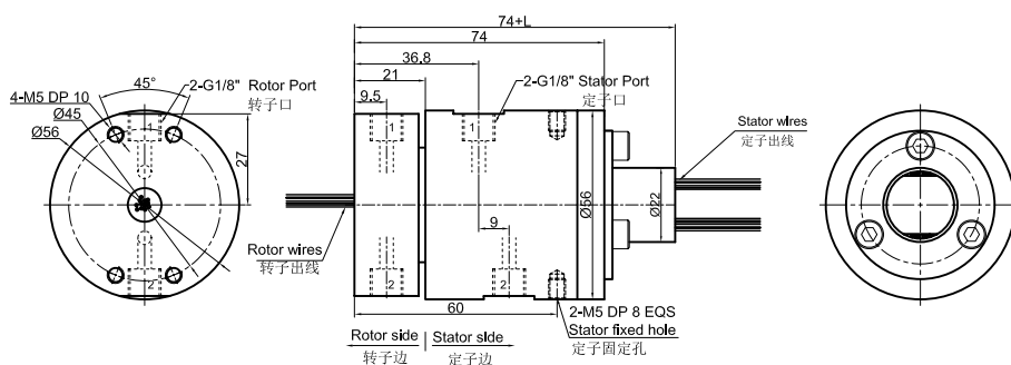
MK21S-S12(S18,S24,S36) 尺寸图 2进2出G1/8"牙+12~36路信号(2A)
