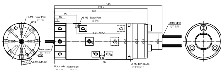
MQR8-S12 尺寸图 8进8出, M5牙 + 12路信号(2A)
