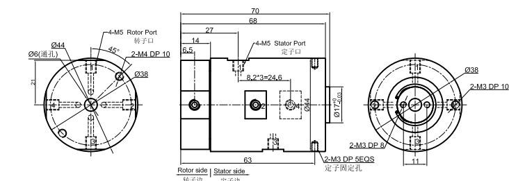
MQR4-S12 尺寸图 4进4出, M5牙 + 12路信号(2A)
