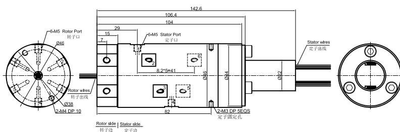
MQR8 尺寸图 8进8出, M5牙
