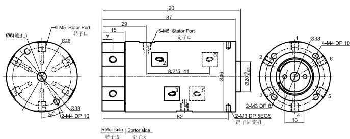
MQR6-S12 尺寸图 6进6出, M5牙 + 12路信号(2A)
