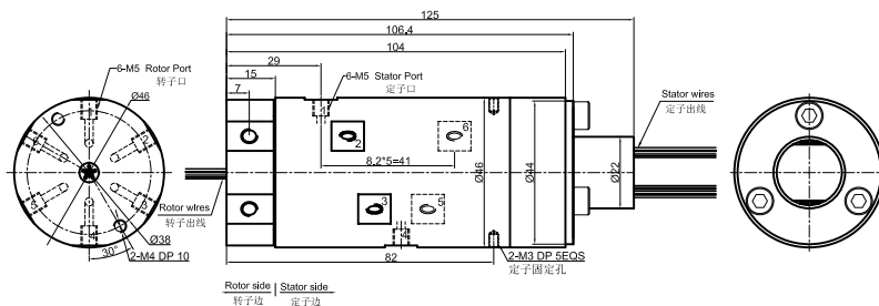
MQR6-S24 尺寸图 6进6出, M5牙 + 24路信号(2A)
