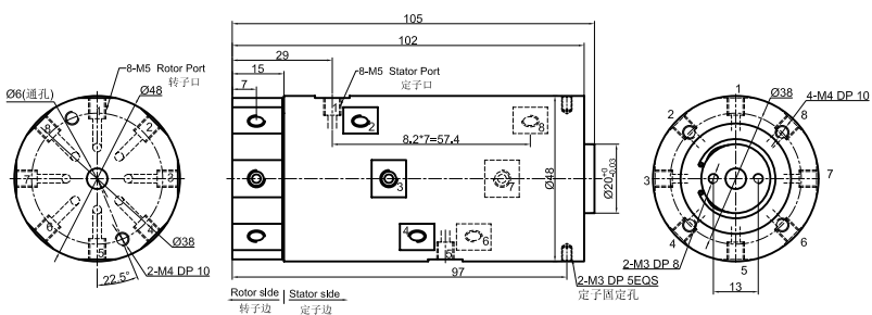
MQR8-S12 尺寸图 8进8出, M5牙 + 12路信号(2A)
