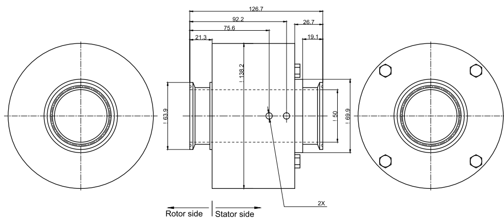
MSCS120 (食品级单路旋转接头) 尺寸图 G2-1/2"牙
