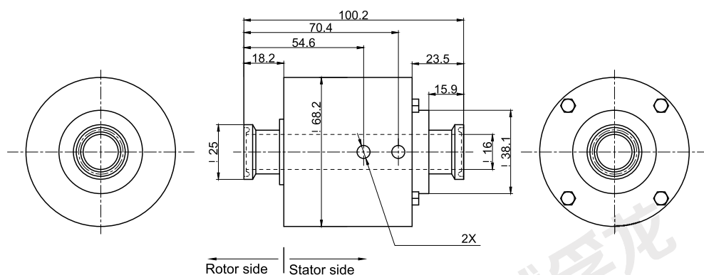
MSCS18 (食品级单路旋转接头) 尺寸图 G1"牙
