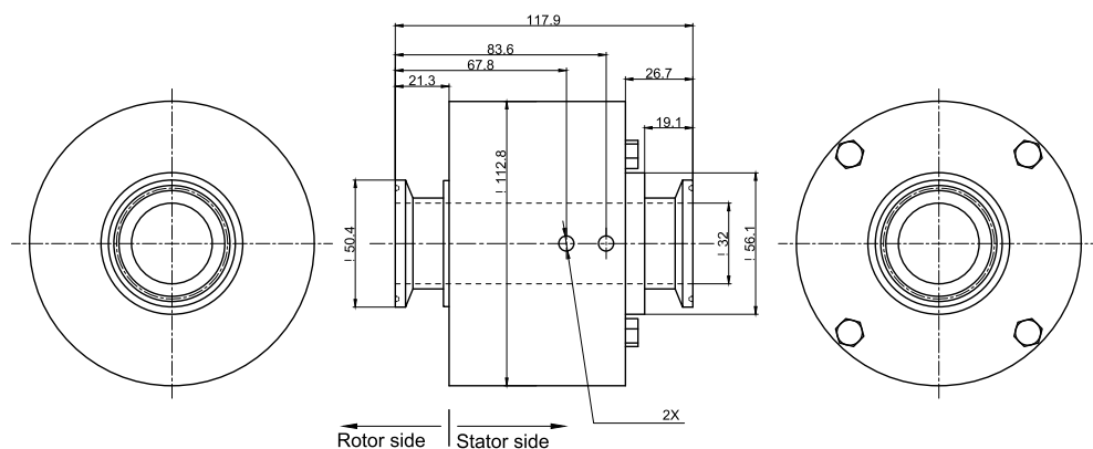
MSCS112 (食品级单路旋转接头) 尺寸图 G1-1/2"牙
