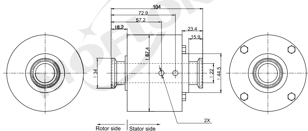
MSCS112 (食品级单路旋转接头) 尺寸图 G1-1/2"牙
