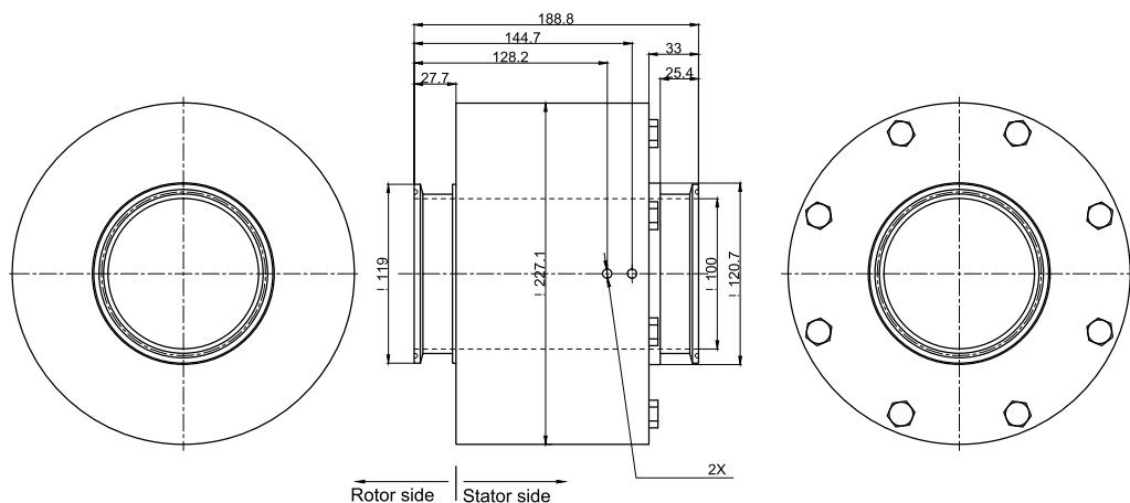
MSCS132（食品级单路旋转接头）尺寸图 G4"牙
