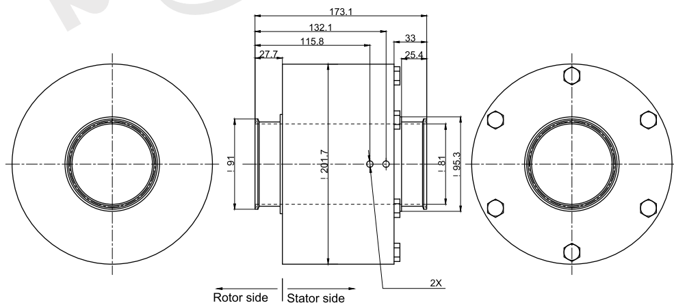
MSCS124 (食品级单路旋转接头) 尺寸图 G3"牙
